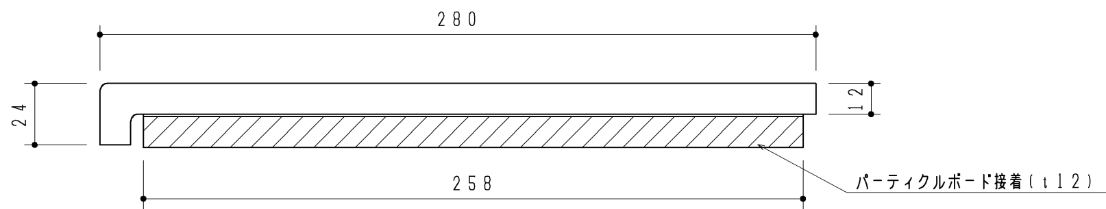
A-A 断面図 (S=1:2)
